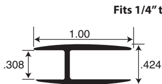
Part # ALUT155-S
