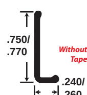
Part # 2163-*
