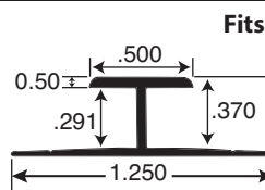
Part # ALU850-*
