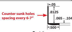
Part # ALU669-*
