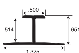
Part # ALU1850-*
