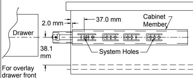
Figure 2 32 mm System—Cabinet
